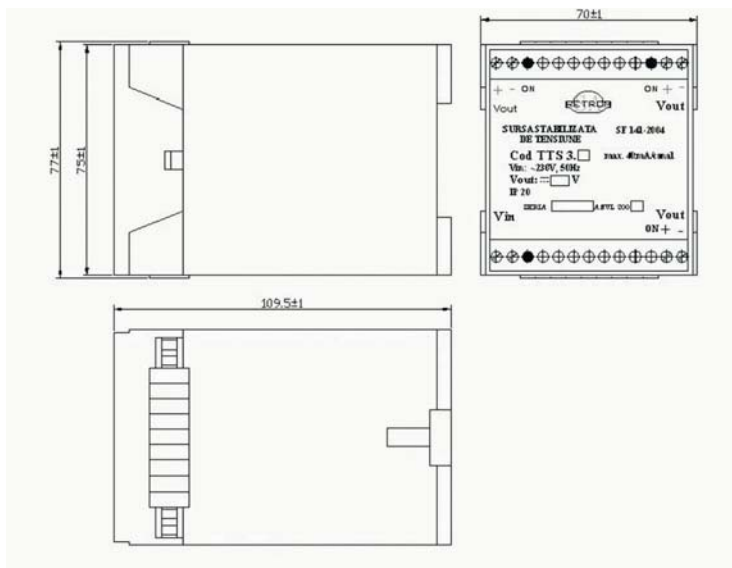
Sursa de tensiune cu două sau trei canale de ieșire Two or three way voltage source
